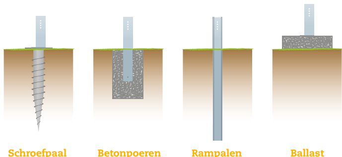
Schroefpaal
